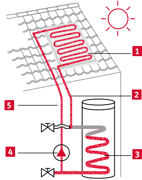
1 Capteur solaire 2 Départ fluide solaire 3 Échangeur ballon 4 Pompe de circulation 5 Arrivée fluide solaire
