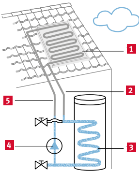
1 Capteur solaire 2 Départ fluide solaire 3 Échangeur ballon 4 Pompe de circulation 5 Arrivée fluide solaire
