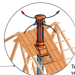
Sortie de toit TRADINOV
